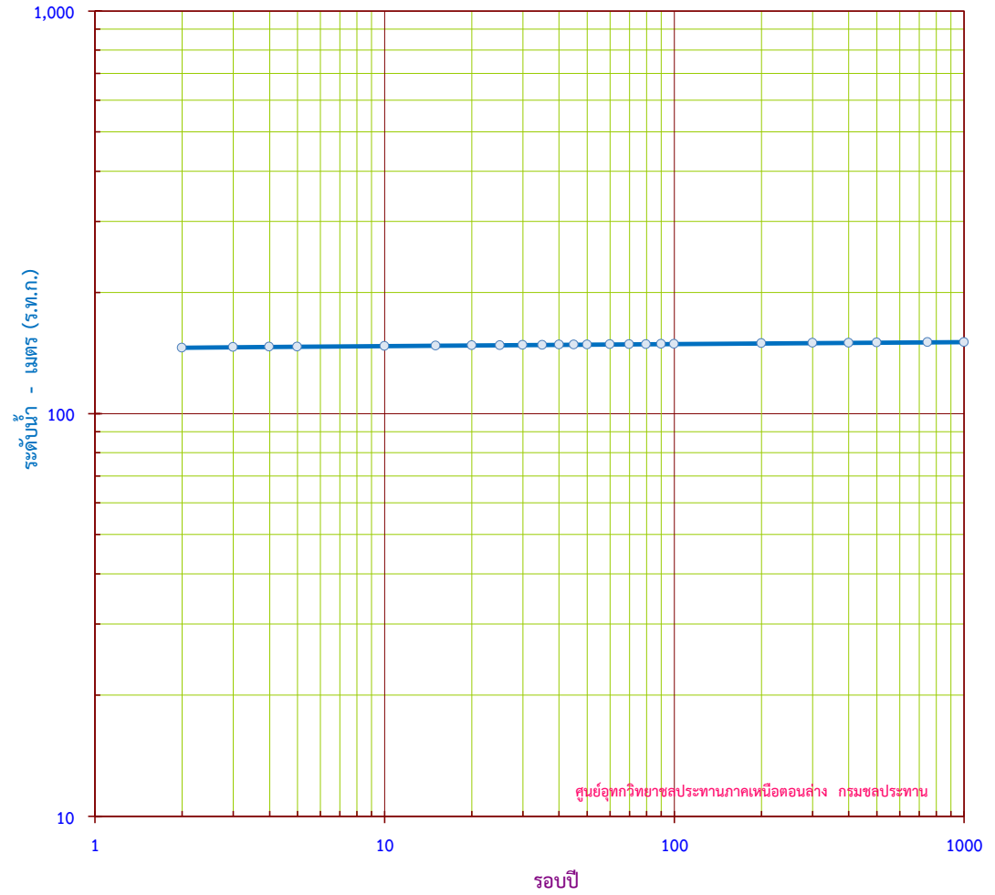
กราฟแสดง ระดับน้ำสูงสุดรายปี ขนาดรอบปีต่างๆ สถานี P.47 อ.คลองลาน จ.กำแพงเพชร
